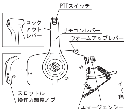
サイドマウントタイプ リモートコントロールボックス仕様
